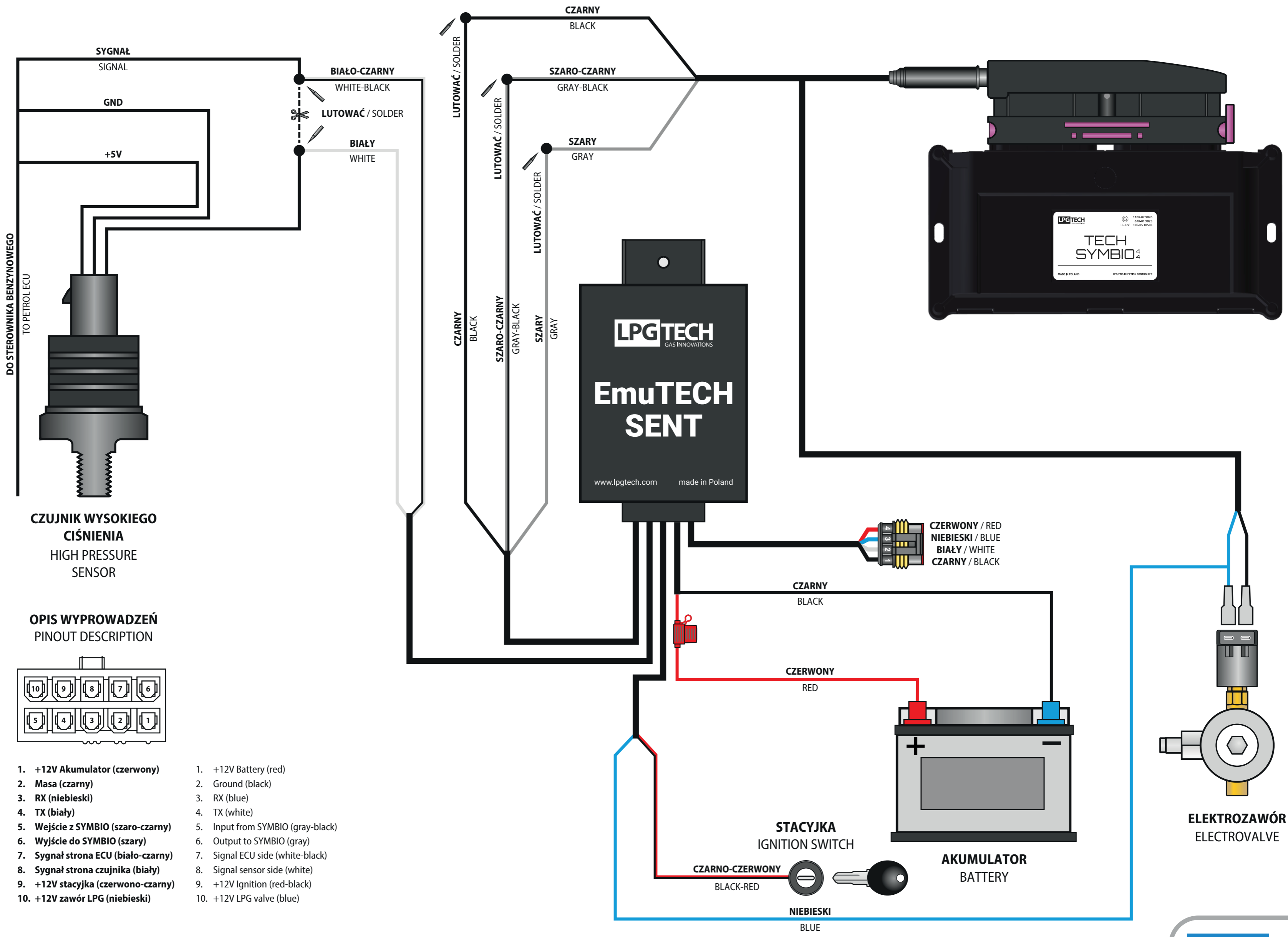
EmuTECH SENT SCHEMAT PODŁĄCZENIA / CONNECTION DIAGRAM
